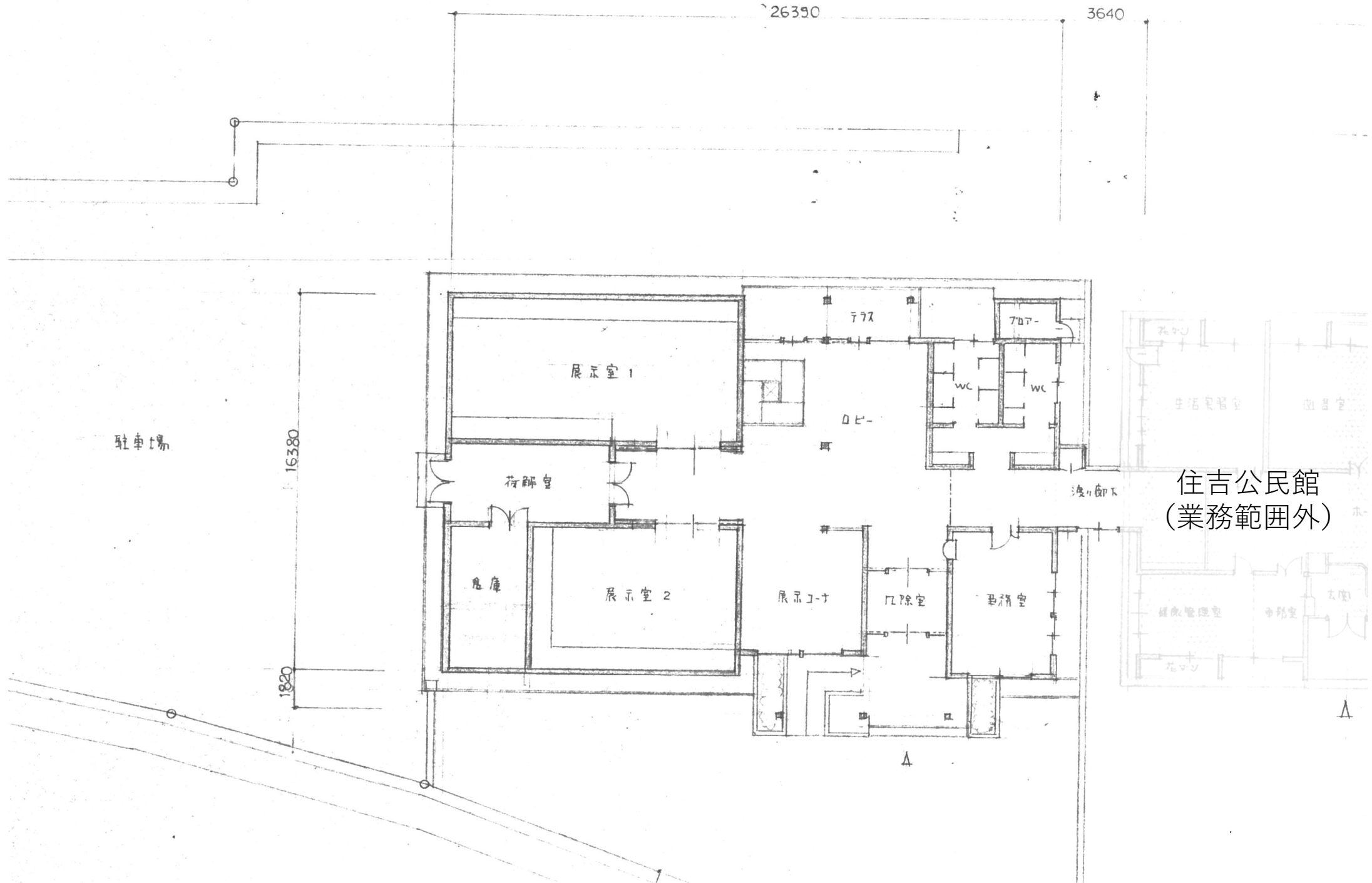
能登中居鋳物館平面図
